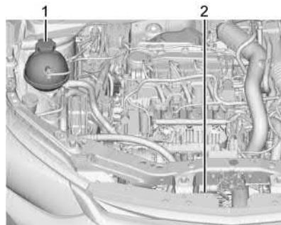
Mostrado o reservatório de expansão do líquido de arrefecimento do 1.0L I3 Turbo, outros são similares
